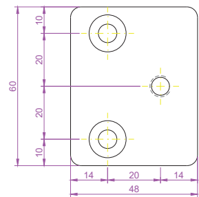
mit versetzter Verschraubung
