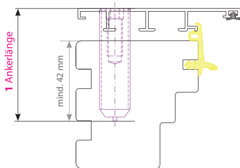
Holz-Aluminiumprofil
