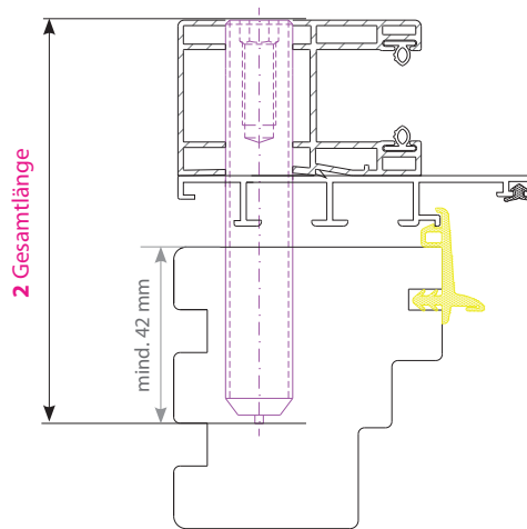
Holz-Aluminiumprofil mit Rolladenführung
