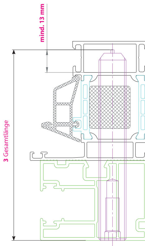
Aluminiumprofil mit Rollladenführung
