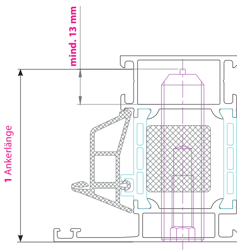
Aluminiumprofil
